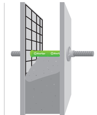
PASO 4: Adaptable a los diferentes grosores de muro
