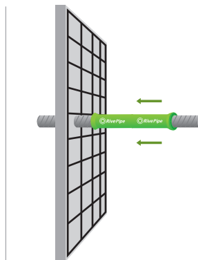
PASO 2: RivePipe protege las varillas o espadines del hormigón cuando se insertan entre los paneles
